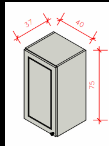
Módulo 05 – Armário Aéreo – 40cm
