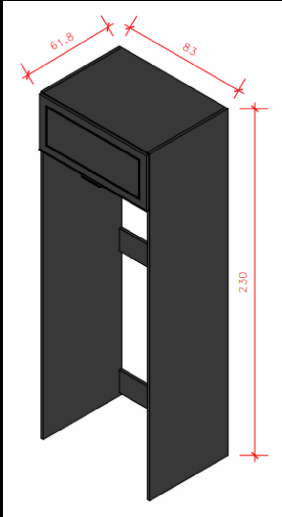
Módulo 08 – Nicho Geladeira com basculante - 83cm
