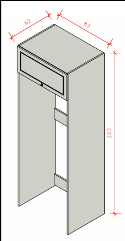
Módulo 08 – Nicho Geladeira com basculante - 83cm
