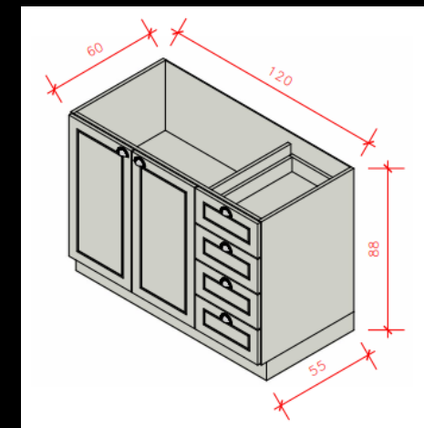
Módulo 06 – Balcão 02 Portas c/ 04 Gavetas - 120cm
