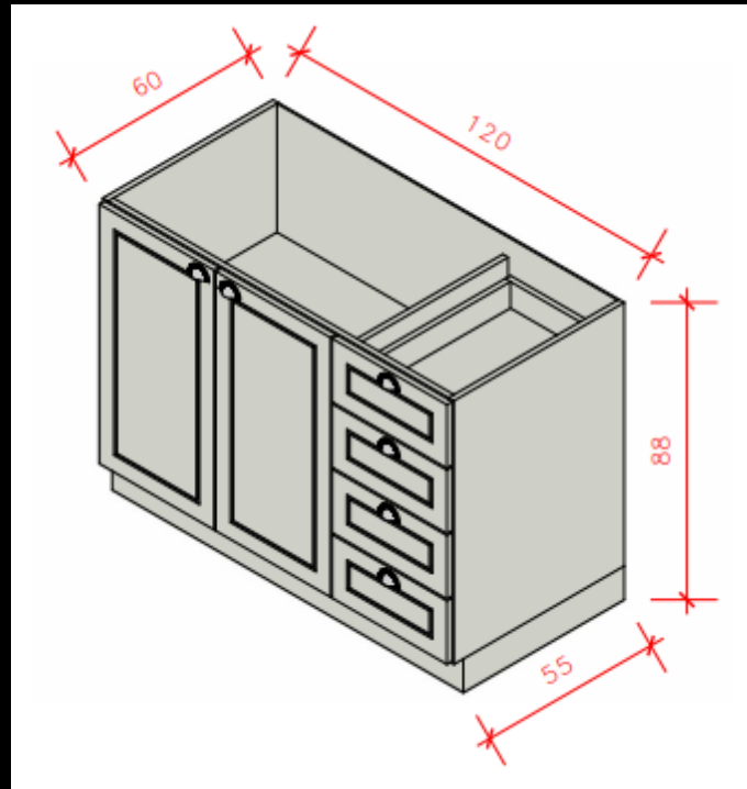
Módulo 08 – Balcão 02 Portas c/ 04 Gavetas - 120cm
