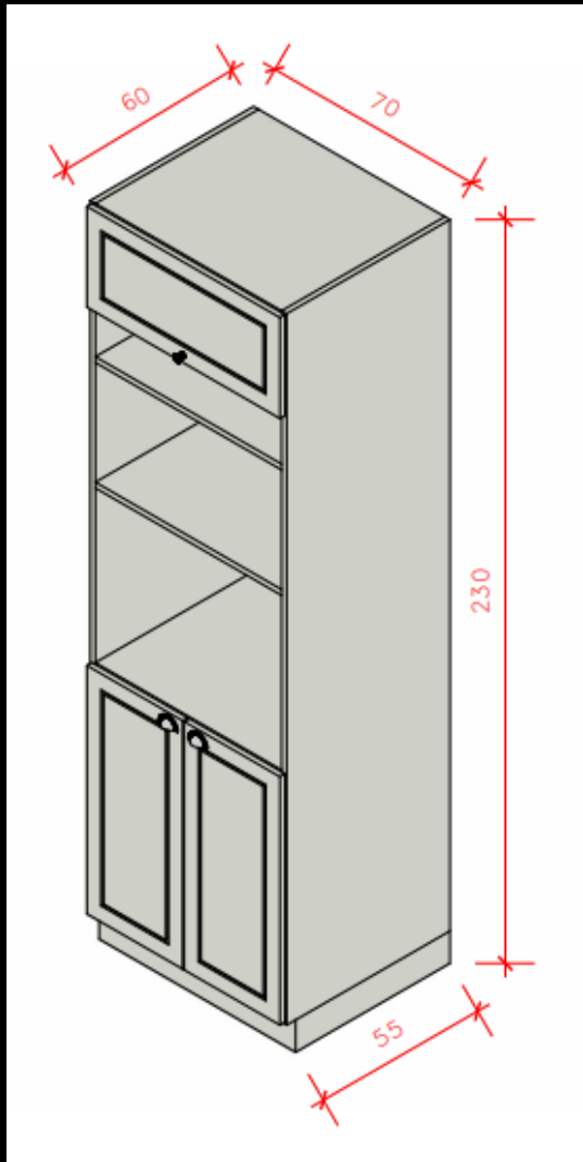
Módulo 01 – Torre fornos 02 Portas c/ 01 Basculante - 70cm – Com fundo e recortes para tomadas.
