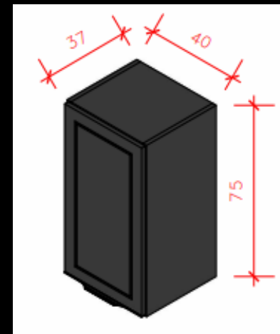
Módulo 05 – Armário Aéreo – 40cm
