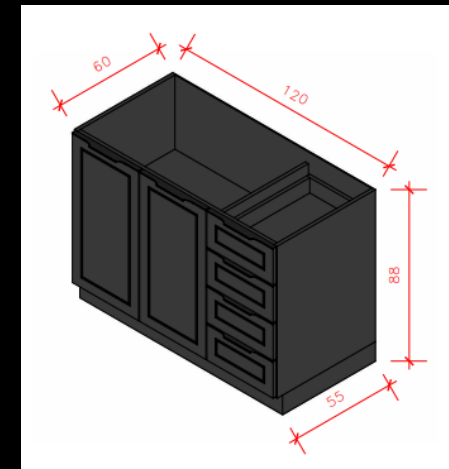
Módulo 06 – Balcão 02 Portas c/ 04 Gavetas - 120cm
