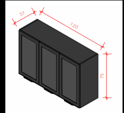
Módulo 07 – Armário aéreo 3 portas de vidro – 120cm
