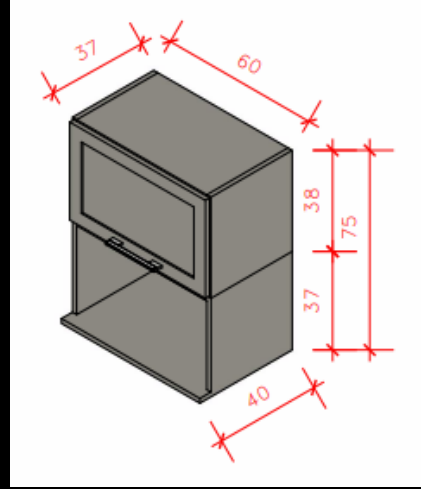
Módulo 02 – Armário superior c/ nicho – 60cm
