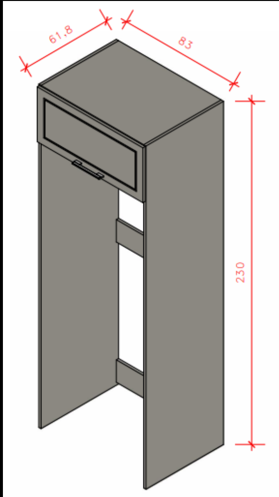
Módulo 08 – Nicho Geladeira com basculante - 83cm
